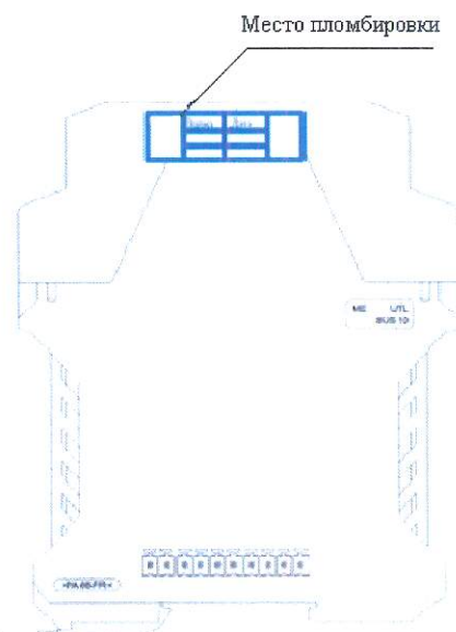
Рисунок 3 – Схемы пломбировки от несанкционированного доступа
